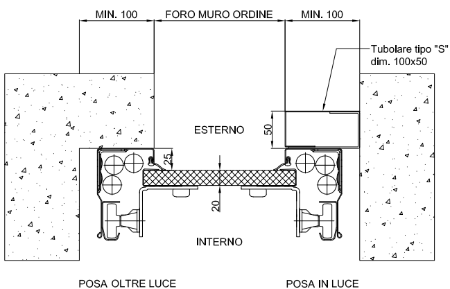
Sezione orizzontale
