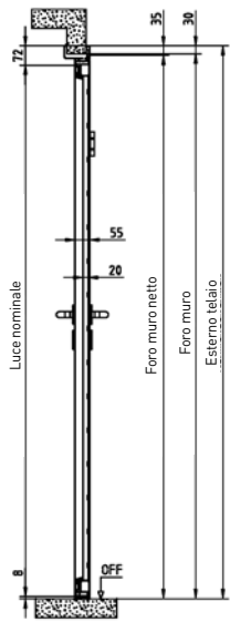
Sezione verticale
