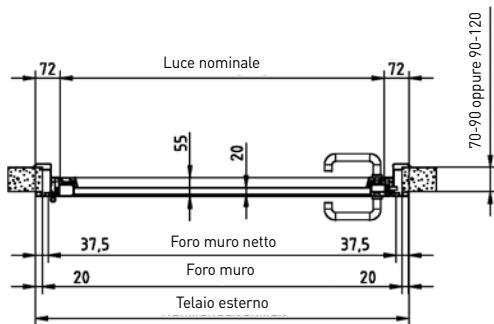
Sezione orizzontale
