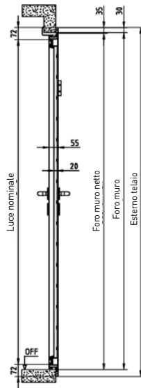
Sezione verticale
